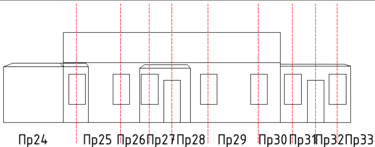
Д-Фасад 2 (фундамент 2, стена 2, покрытие 2)
