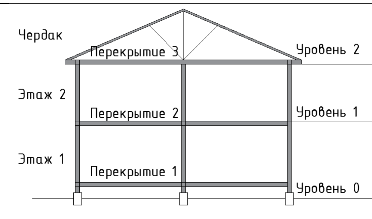
Схема разреза
