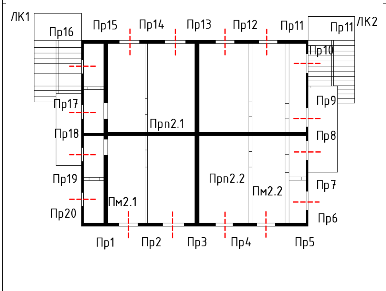
План 2-ого этажа
