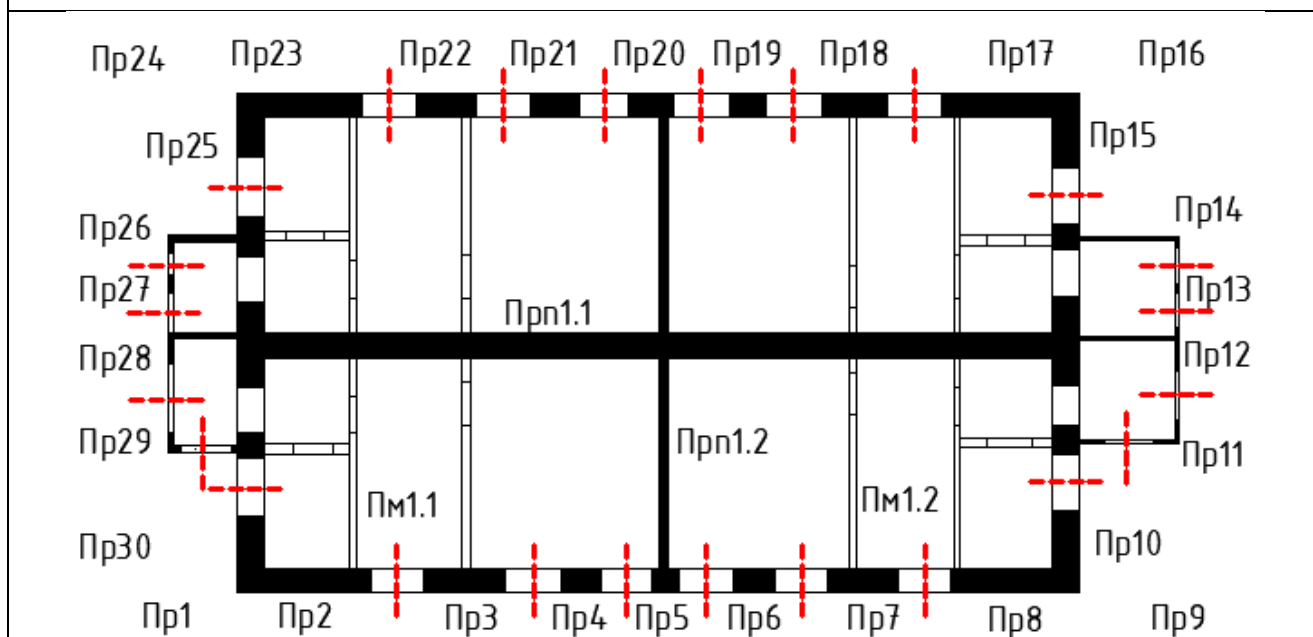
План 2-ого этажа
