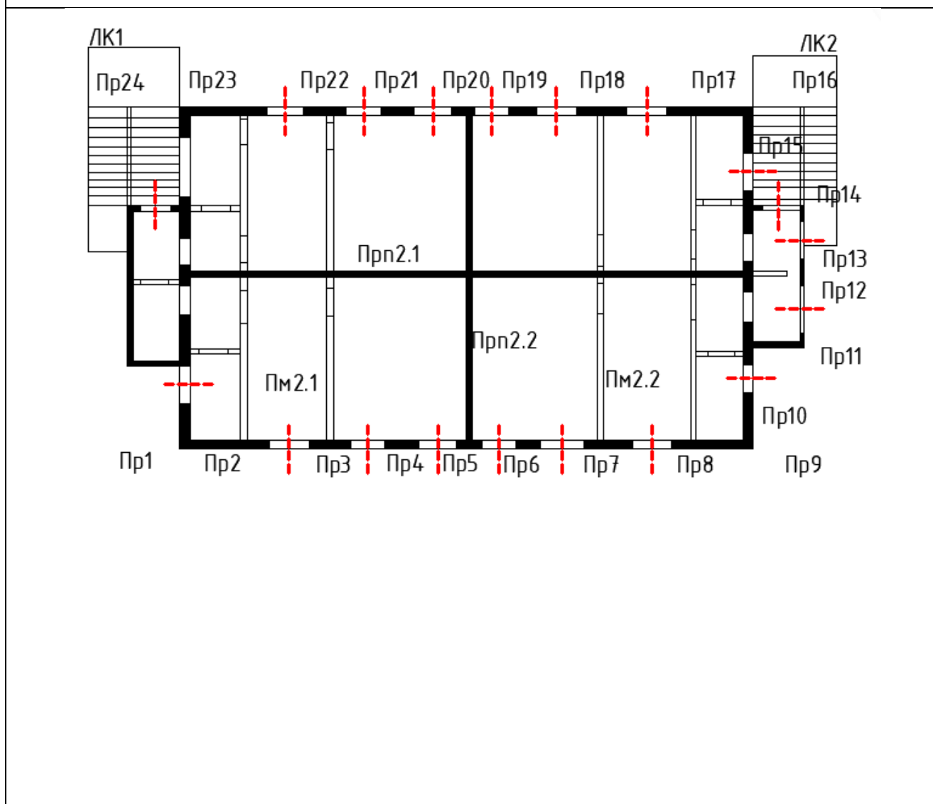
План 2-ого этажа
