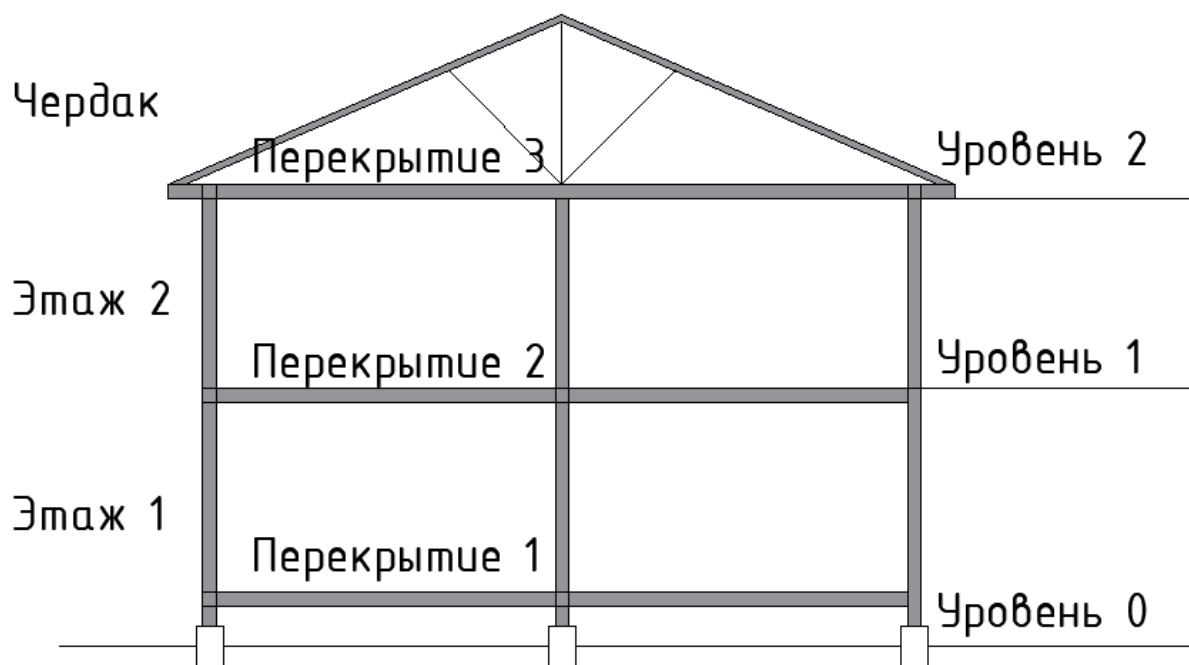
Схема разреза
