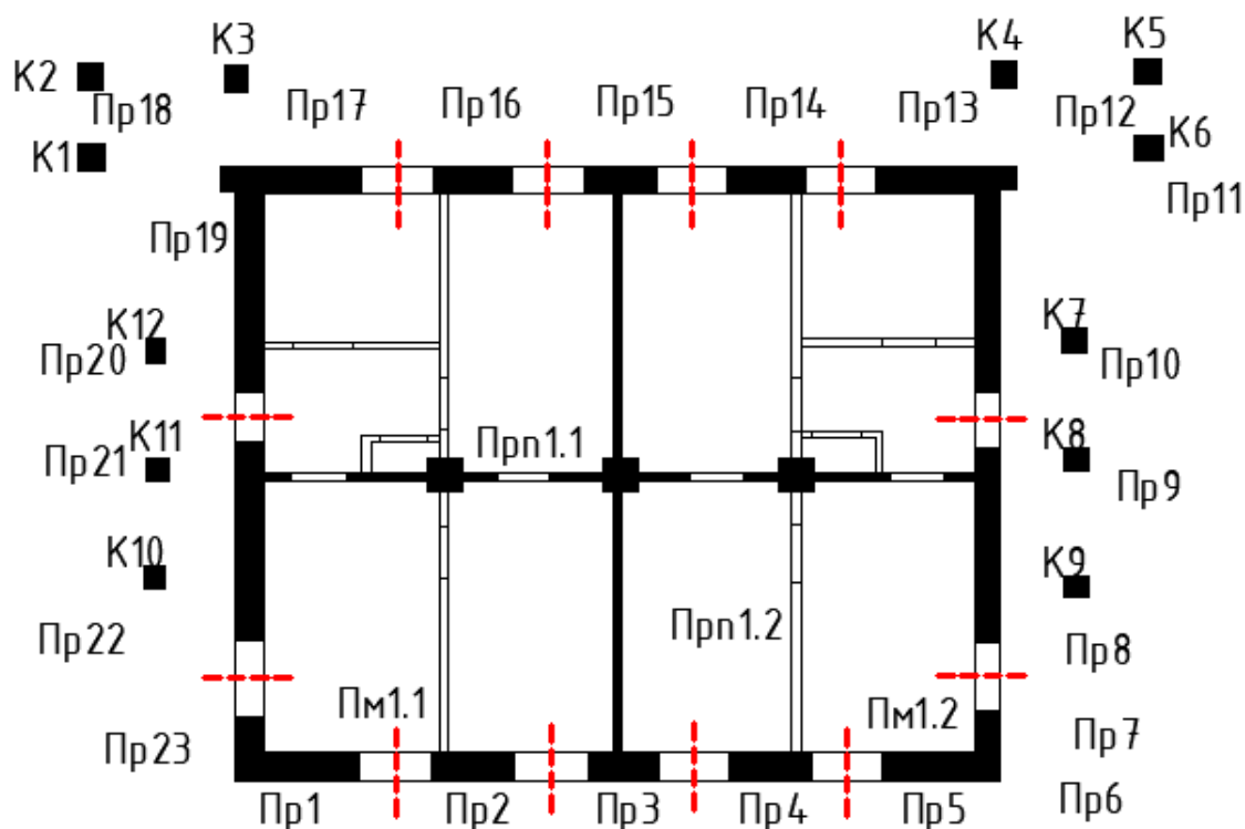
План 2-ого этажа
