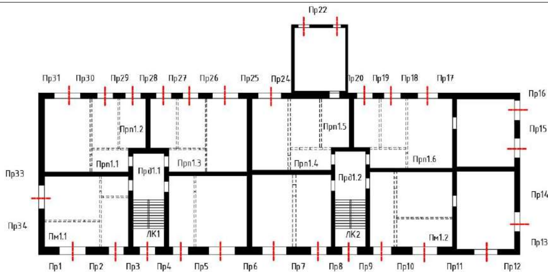
План 2-ого этажа
