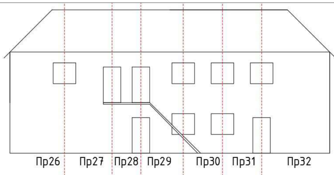
Фасад 1 (фундамент 1, стена 1, покрытие 1) (литер Г)
