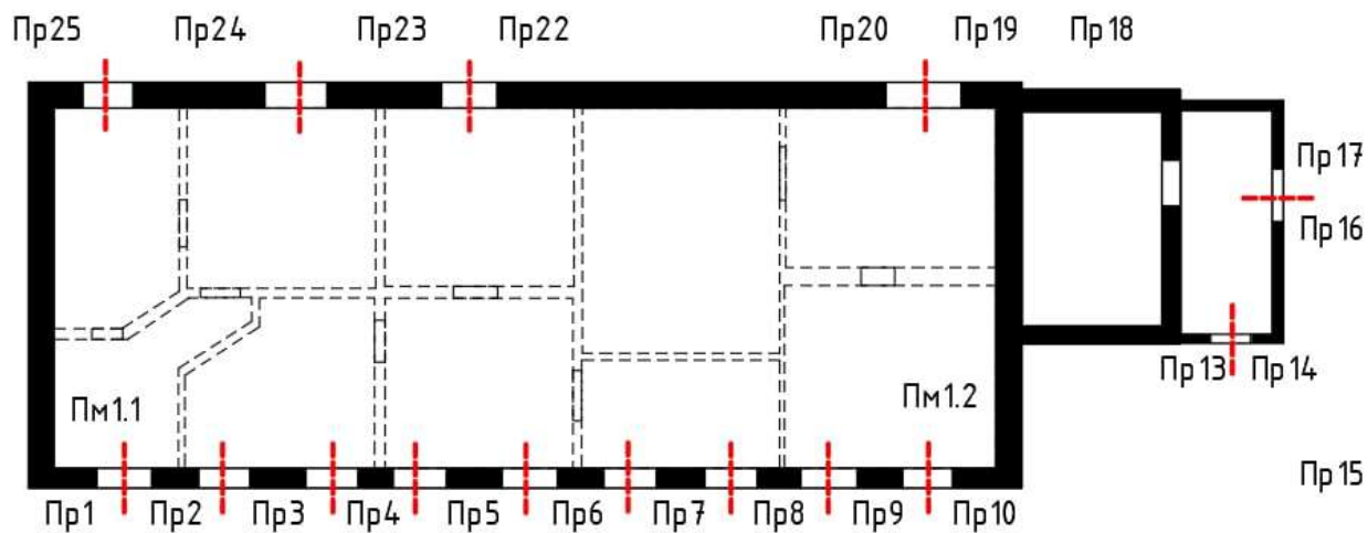
План 2-ого этажа (литер Б)
