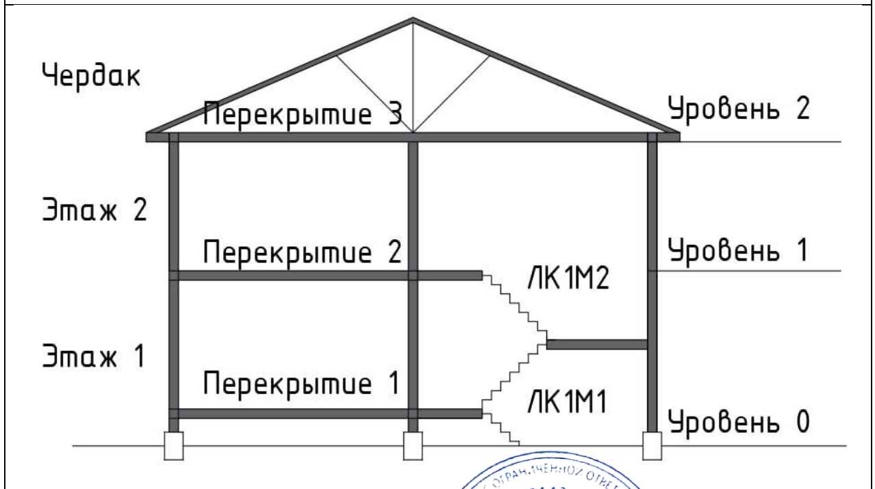
Схема разреза
