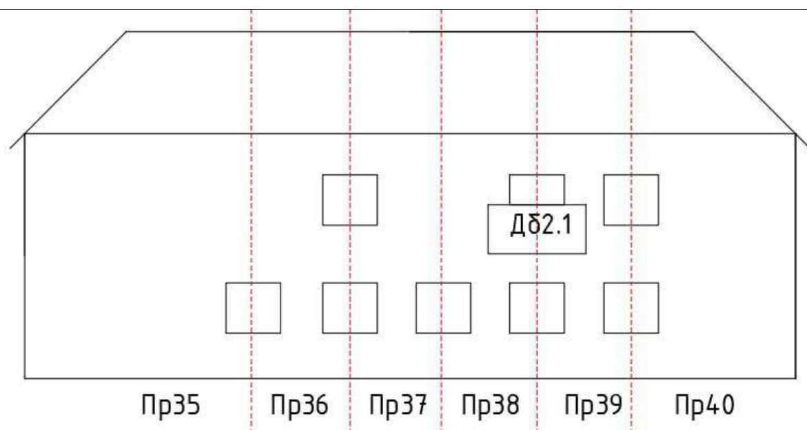
Фасад 3 (фундамент 3, стека 3, покрытие 3) (литер Г)
