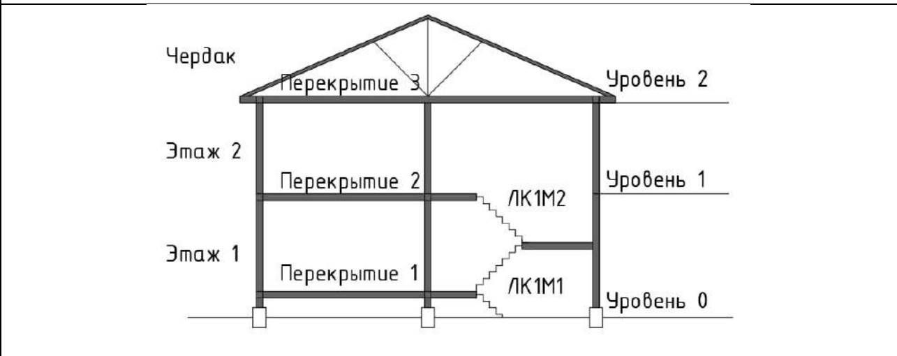
Схема разреза
