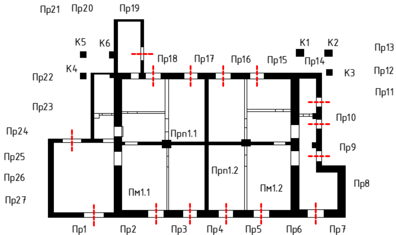
План 1-ого этажа
