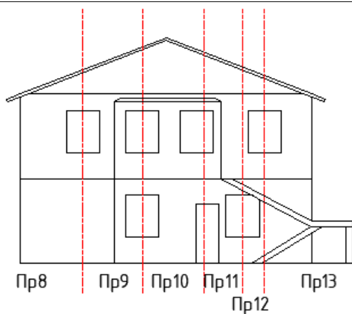
Фасад 3 (фундамент 3, стека 3, покрытие 3)
