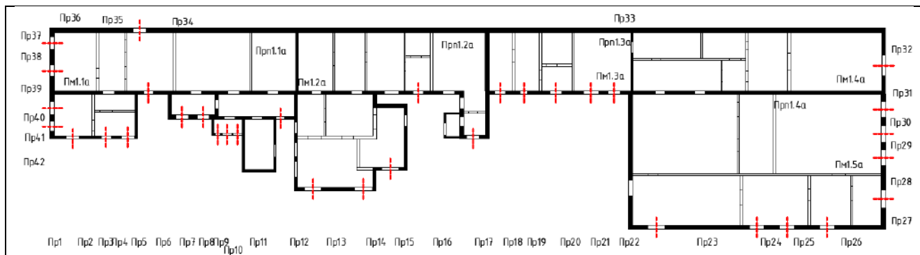
А-План 2-ого этажа
