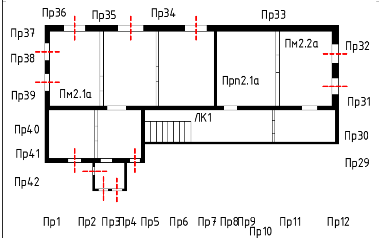
А-Фасад 1 (фундамент 1, стена 1, покрытие 1)
