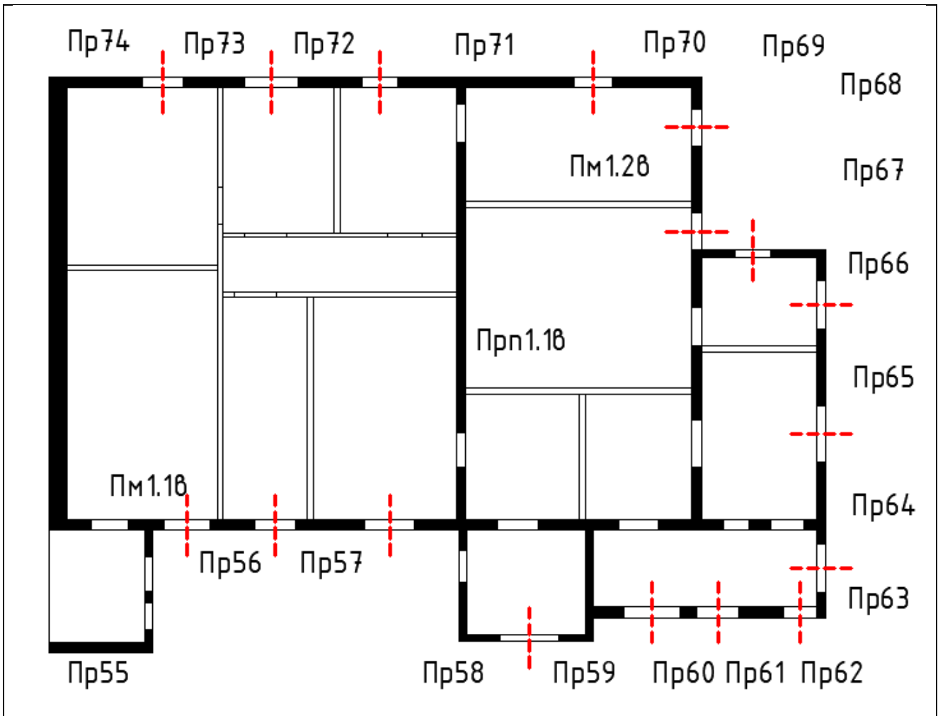
В-Фасад 1 (фундамент 1, стена 1, покрытие 1)
