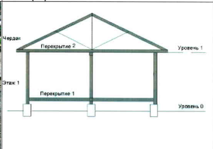
Схема разреза
