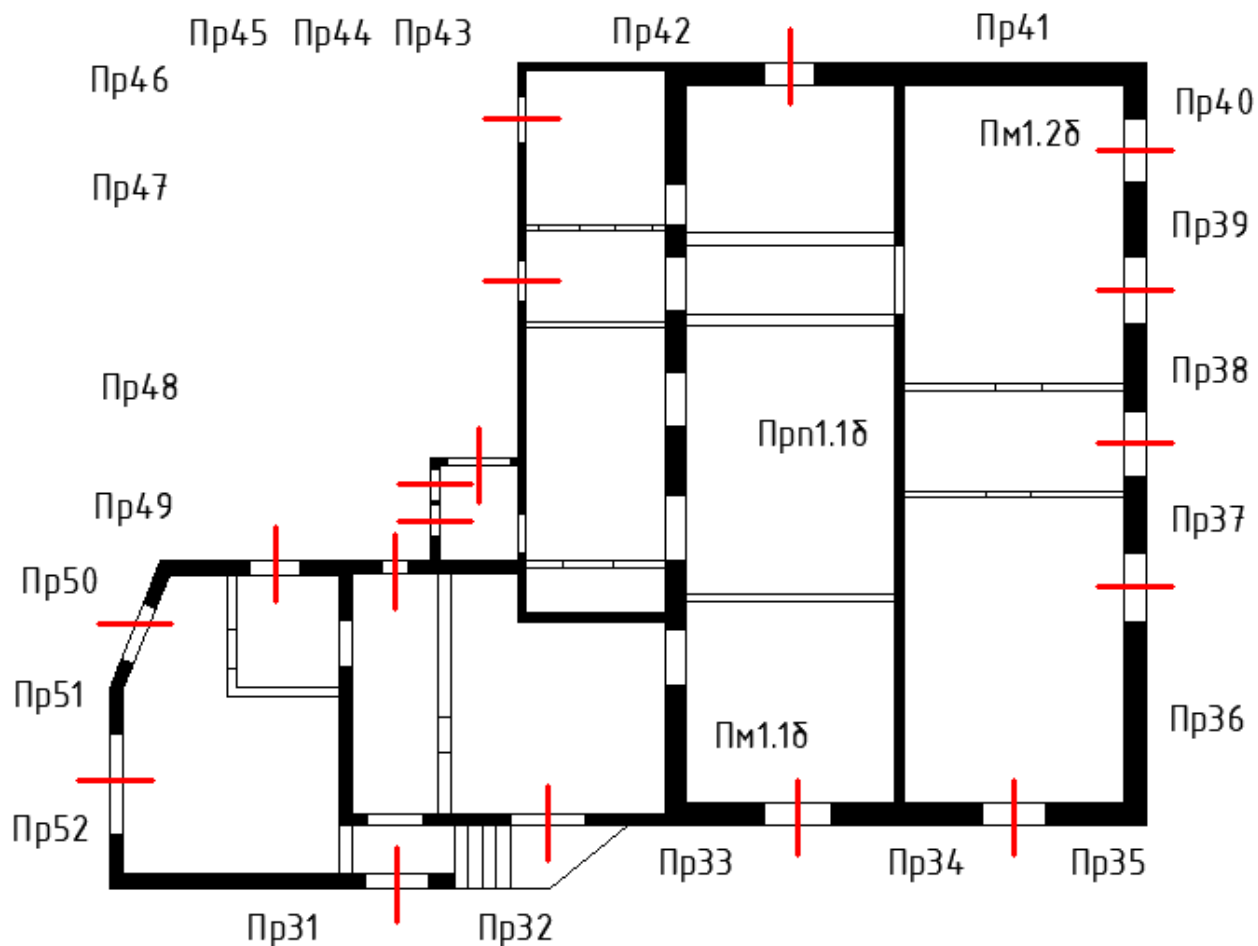
Б-Фасад 1 (фундамент 1, стена 1, покрытие 1)
