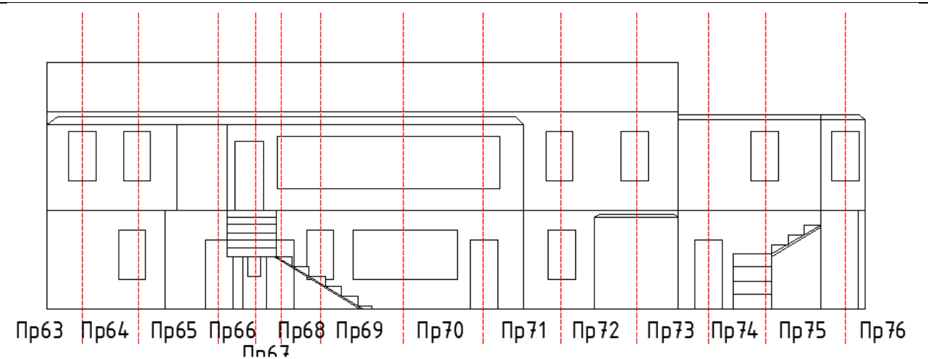
Г-Фасад 2 (фундамент 2, стена 2, покрытие 2)
