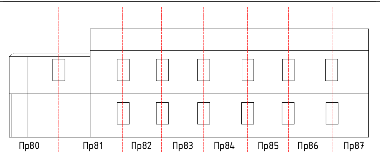
Г-Фасад 3 (фундамент 3, стена 3, покрытие 3)
