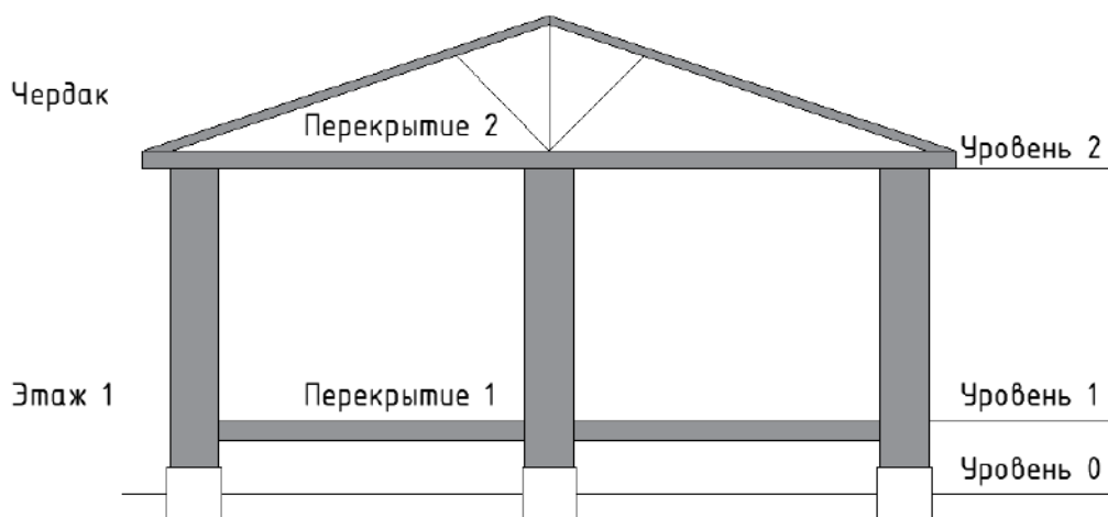
А,Б,В-Схема разреза
