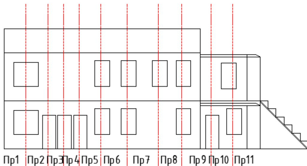
Фасад 1 (фундамент 1, стена 1, покрытие 1)
