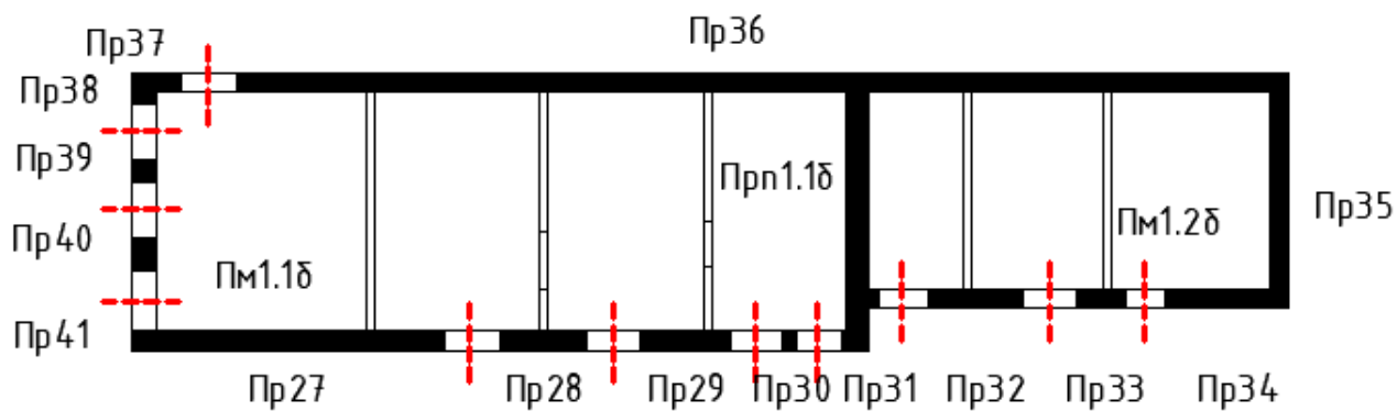
Б-Фасад 1 (фундамент 1, стена 1, покрытие 1)
