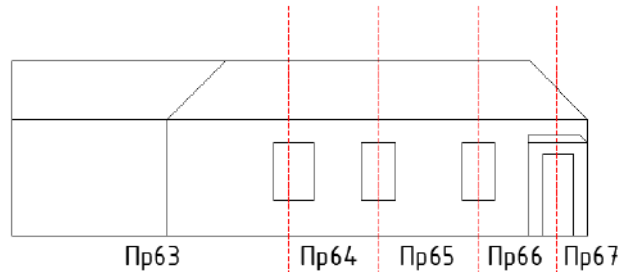
Г-Фасад 4 (фундамент 4, стека 4, покрытие 4)
