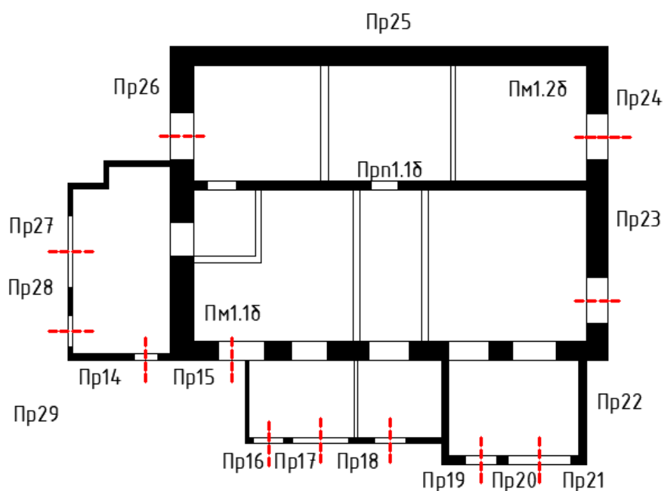
Б-Фасад 1 (фундамент 1, стена 1, покрытие 1)
