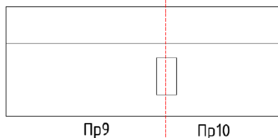
Фасад 4 (фундамент 4, стена 4, покрытие 4)
