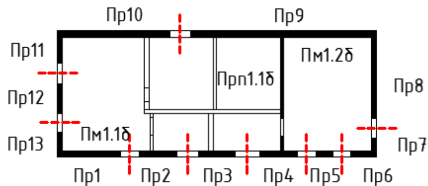
Фасад 1 (фундамент 1, стена 1, покрытие 1)
