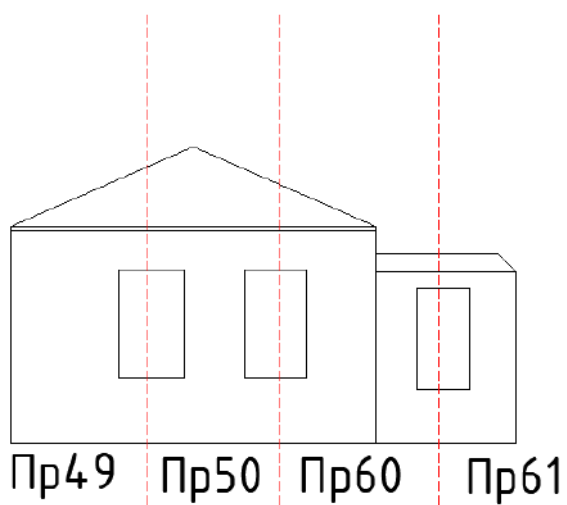
Г-Фасад 1 (фундамент 1, стена 1, покрытие 1)
