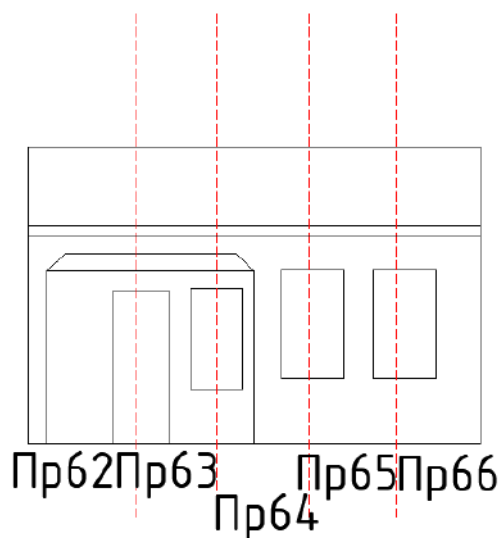
Г-Фасад 4 (фундамент 4, стена 4, покрытие 4)
