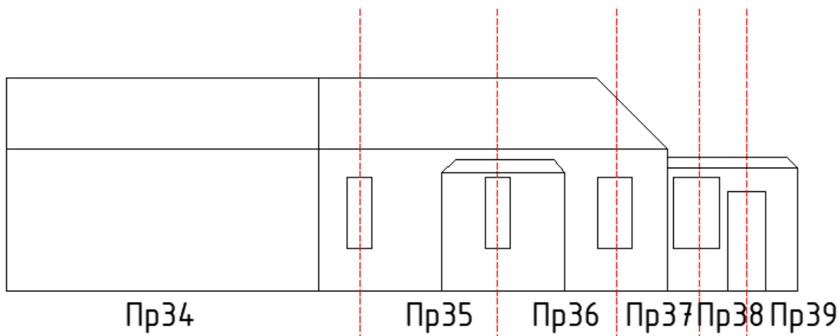
В-Фасад 2 (фундамент 2, стена 2, покрытие 2)
