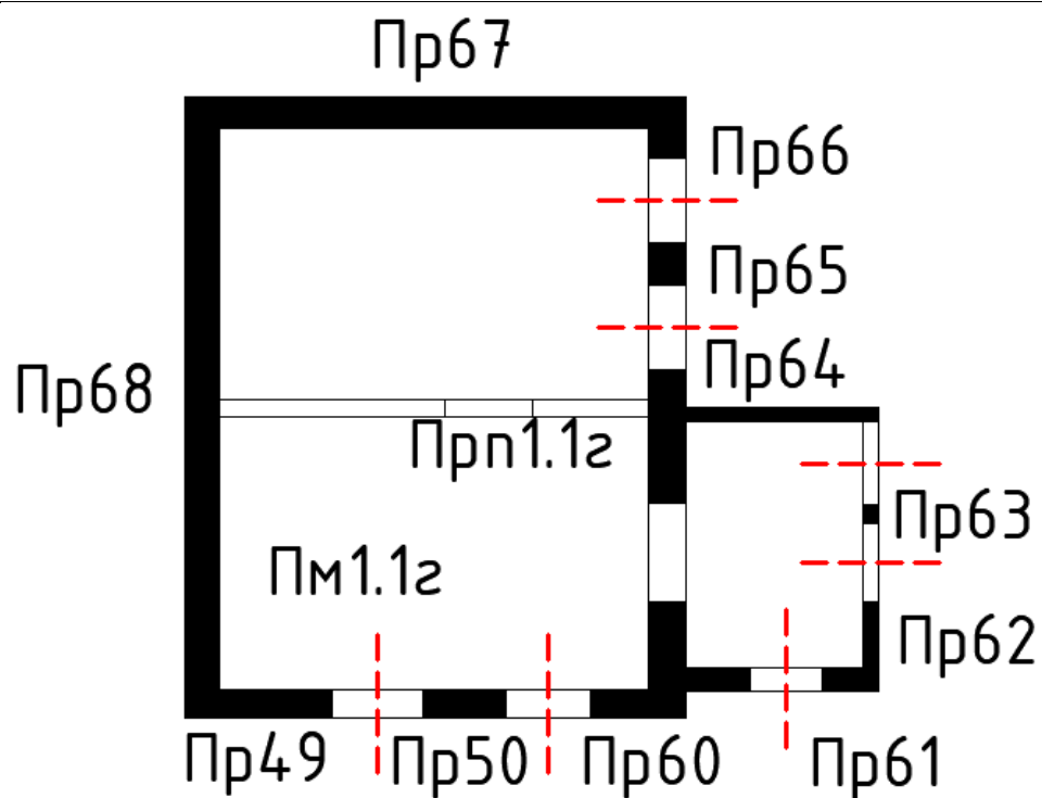
Г-Фасад 1 (фундамент 1, стена 1, покрытие 1)
