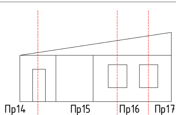
А-Фасад 4 (фундамент 4, стена 4, покрытие 4)
