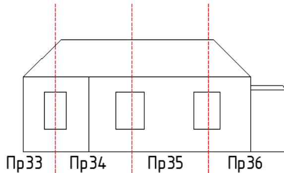
А-Фасад 4 (фундамент 4, стена 4, покрытие 4)
