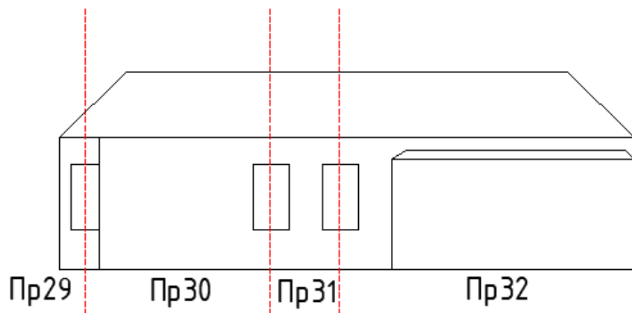
А-Фасад 3 (фундамент 3, стена 3, покрытие 3)
