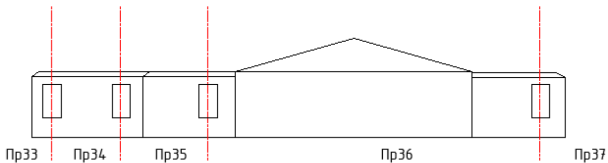
Б-Фасад 4 (фундамент 4, стена 4, покрытие 4)
