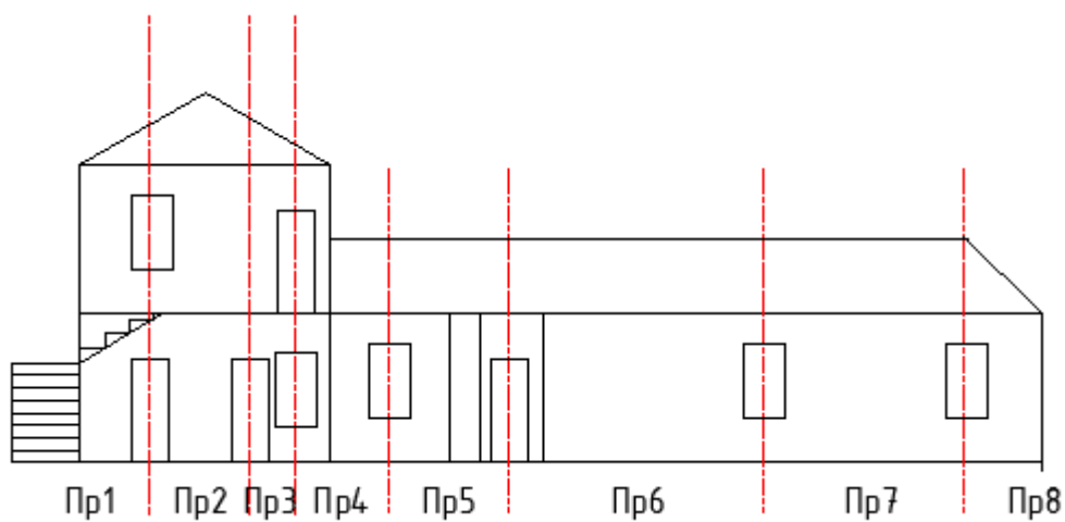
А-Фасад 1 (фундамент 1, стена 1, покрытие 1)
