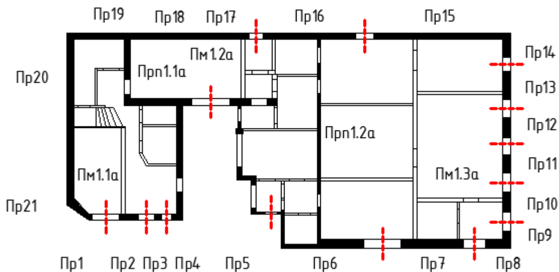
А-План 2-ого этажа
