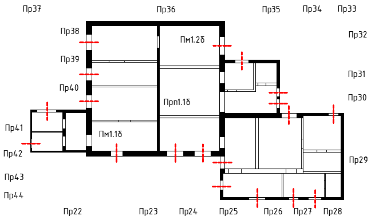
Б-План 1-ого этажа
