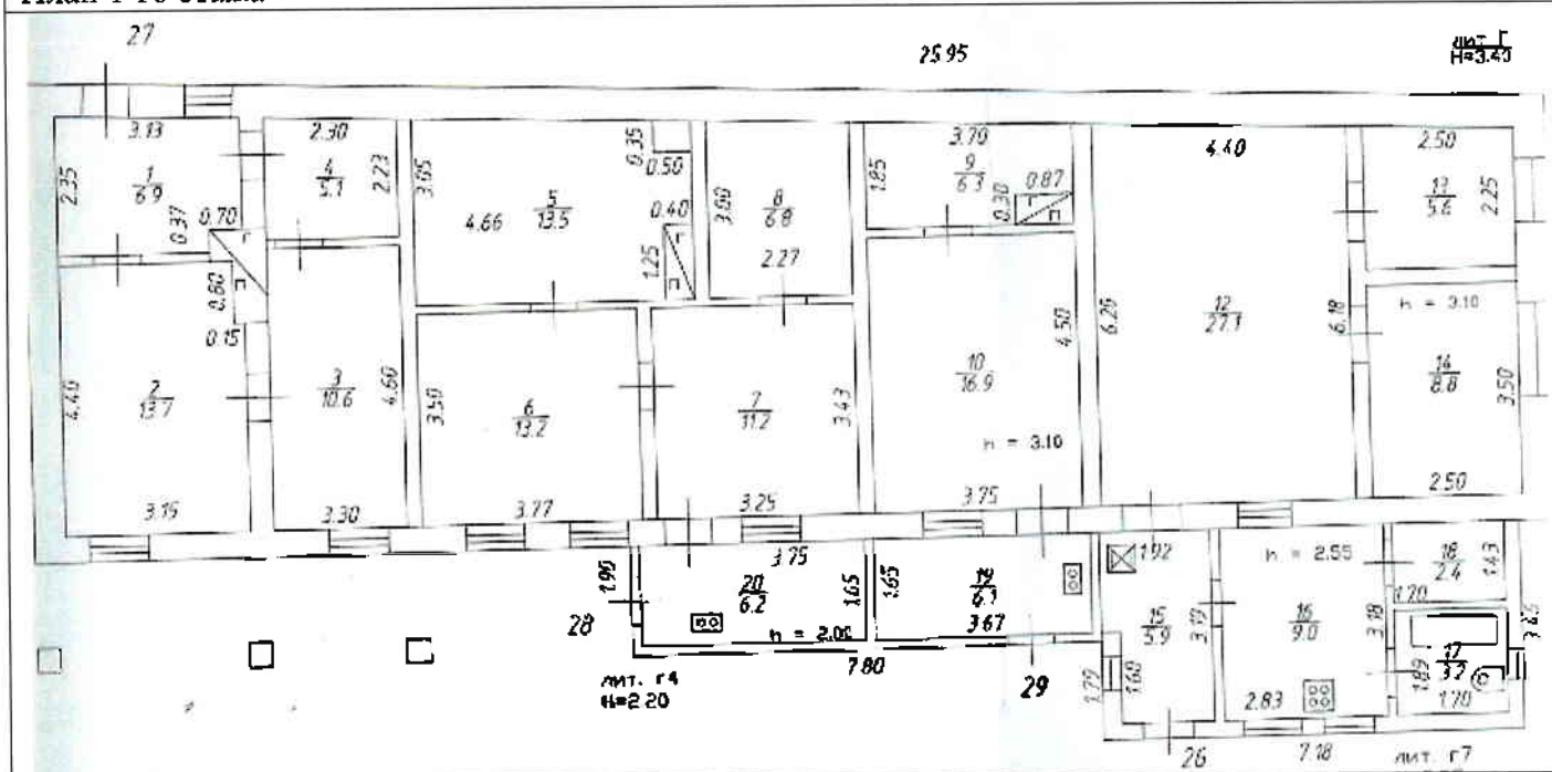
План 1-го этажа
