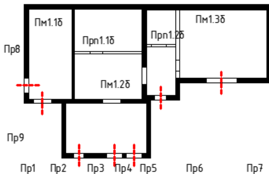
Б-Фасад 1 (фундамент 1, стена 1, покрытие 1)
