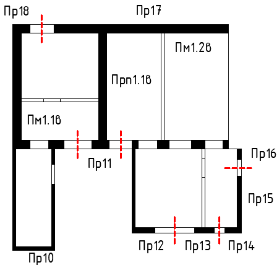
В-Фасад 1 (фундамент 1, стена 1, покрытие 1)
