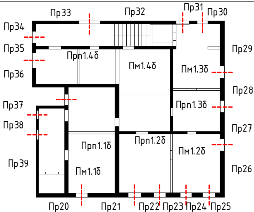
Б-План 1-ого этажа
