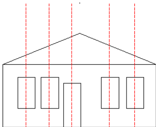
Б-Фасад 1 (фундамент 1, стена 1, покрытие 1)
