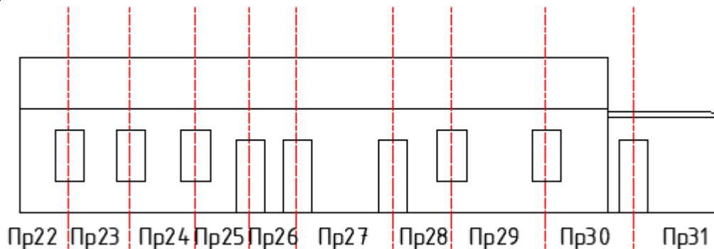
В-Фасад 1 (фундамент 1, стена 1, покрытие 1)
