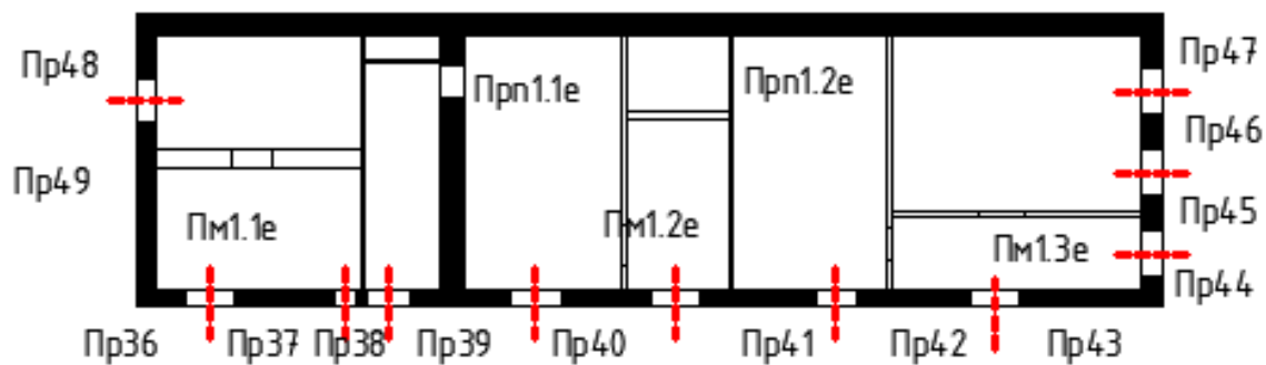
Е-План 1-ого этажа
