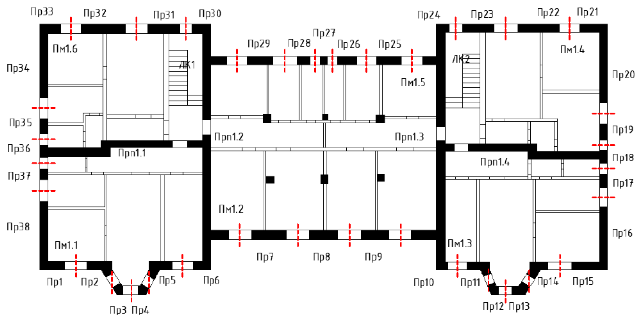
План 2-ого этажа
