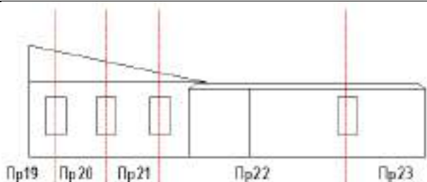
Б-Фасад 1 (фундамент 1, стена 1, покрытие 1)
