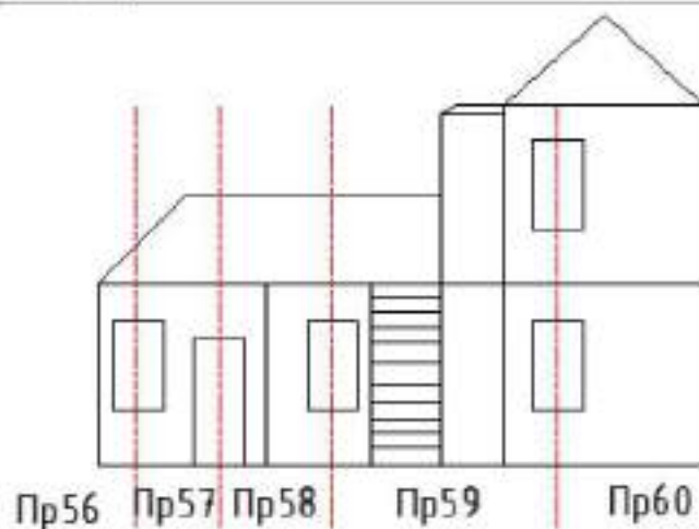
В-Фасад 2 (фундамент 2, стена 2, покрытие 2)
