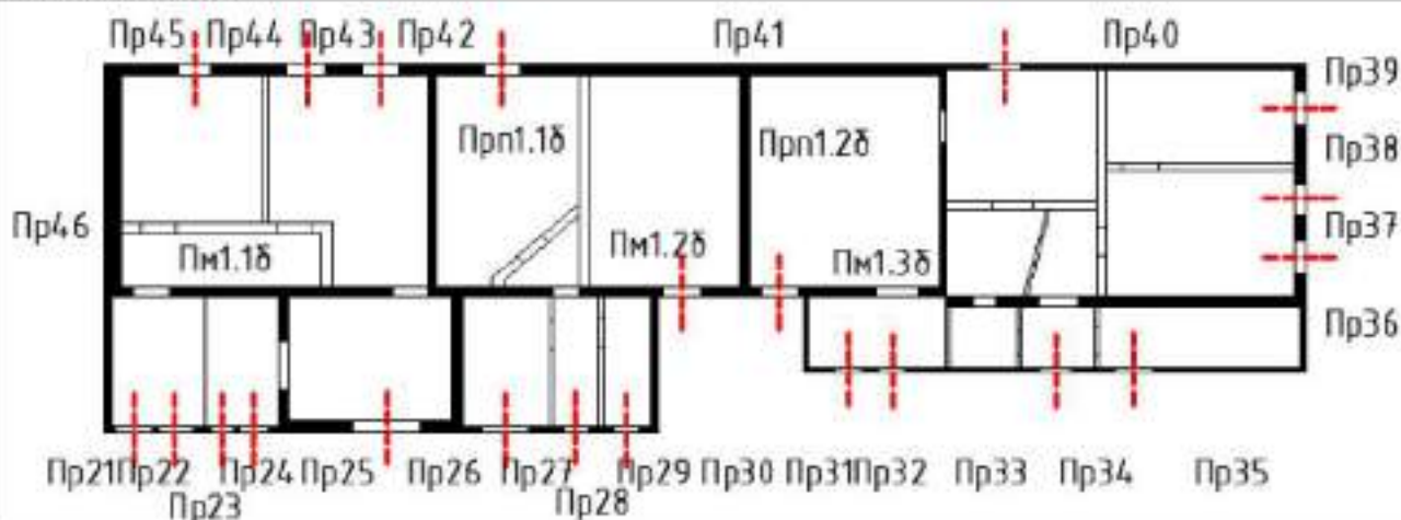
Б-План 1-ого этажа
