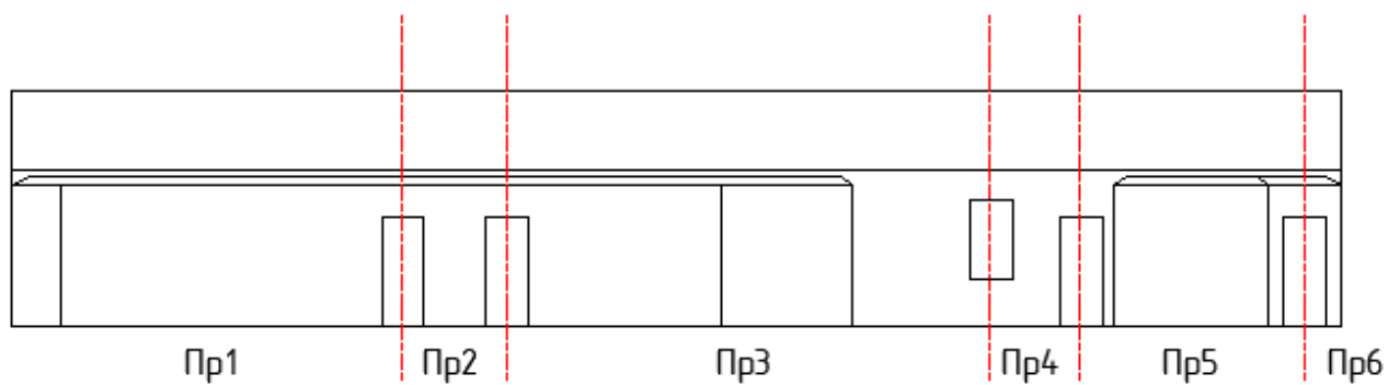
Фасад 2 (фундамент 2, стена 2, покрытие 2)
