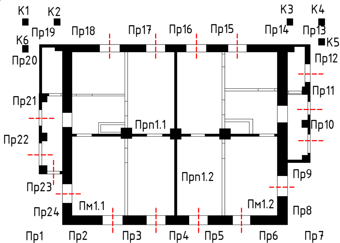
План 1-ого этажа
