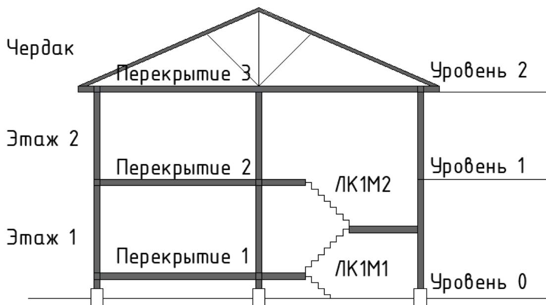
Схема разреза
