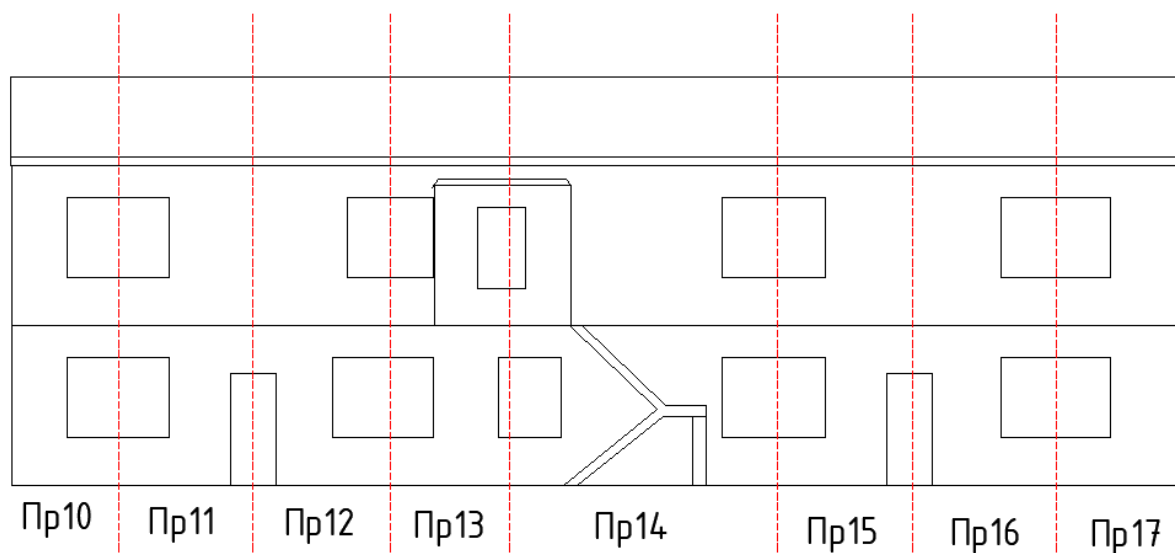
Фасад 3 (фундамент 3, стена 3, покрытие 3)
