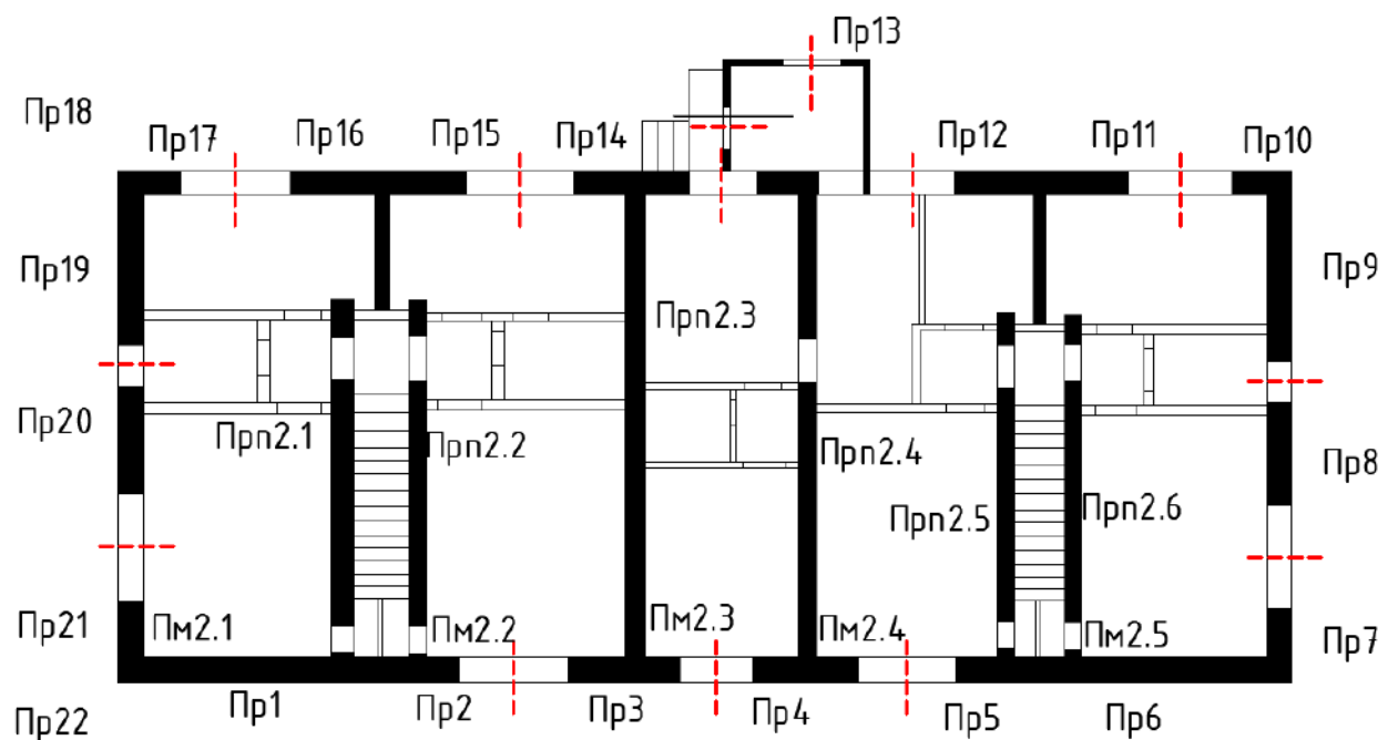
План 2-ого этажа
