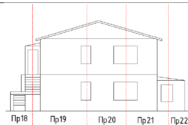
Фасад 4 (фундамент 4, стена 4, покрытие 4)
