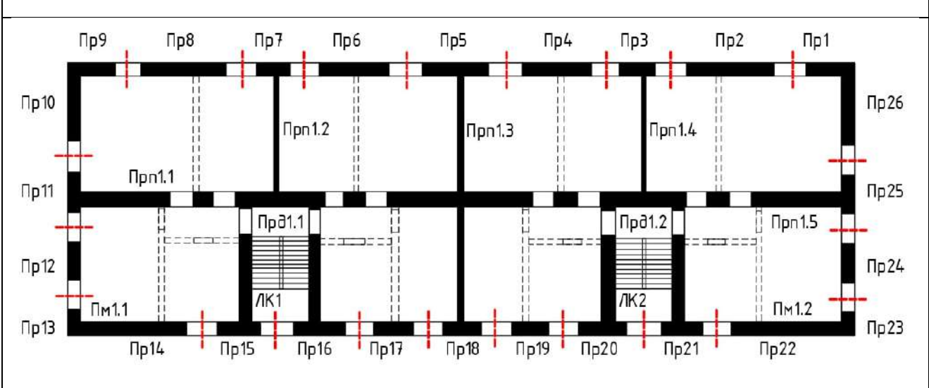
План 2-ого этажа
