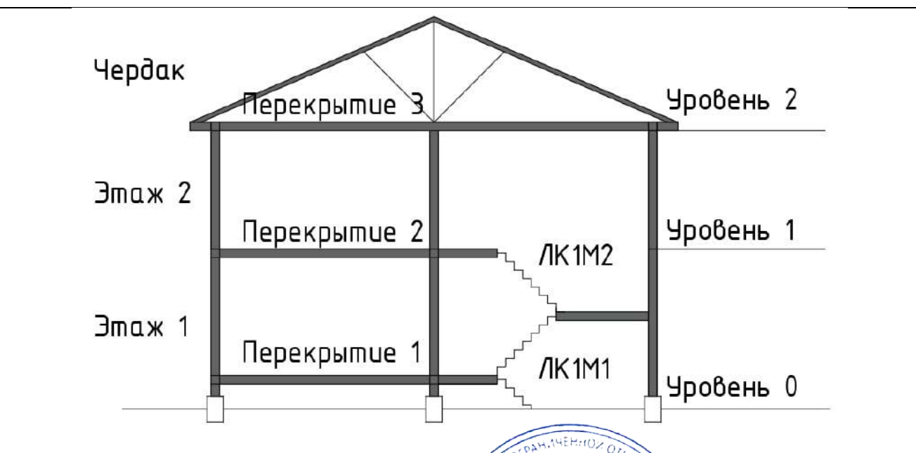
Схема разреза
