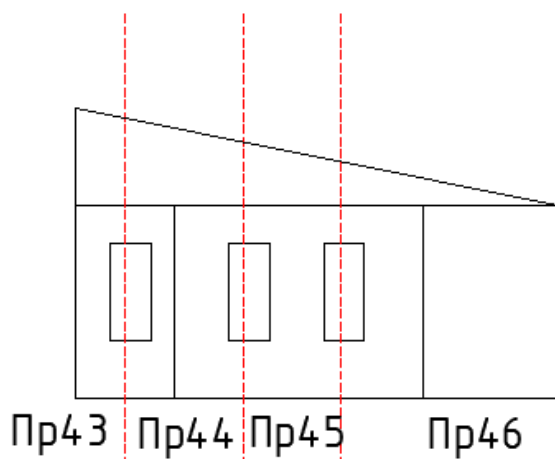
Д-Фасад 3 (фундамент 3, стена 3, покрытие 3)
