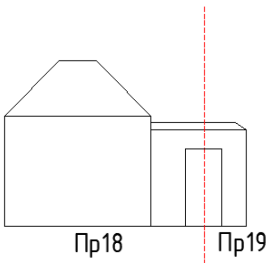
В-Фасад 3 (фундамент 3, стена 3, покрытие 3)
