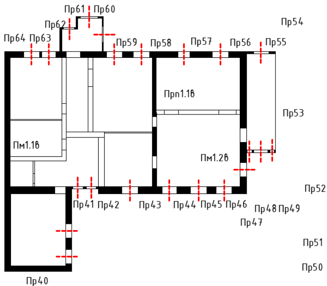
В-План 1-ого этажа
