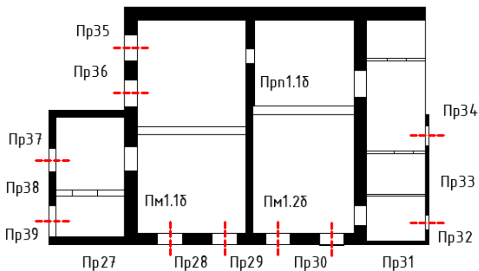
Б-План 1-ого этажа
