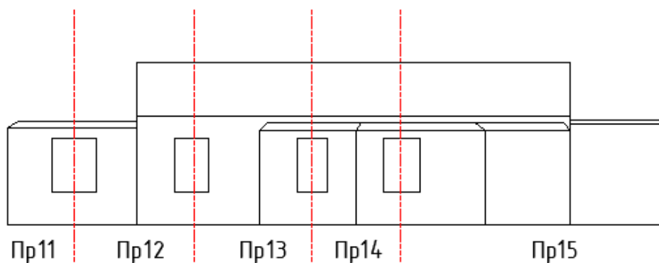
А-Фасад 3 (фундамент 3, стека 3, покрытие 3)
