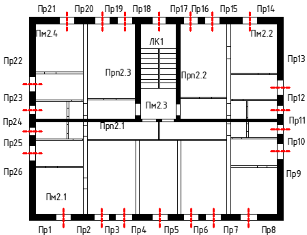
План 2-ого этажа
