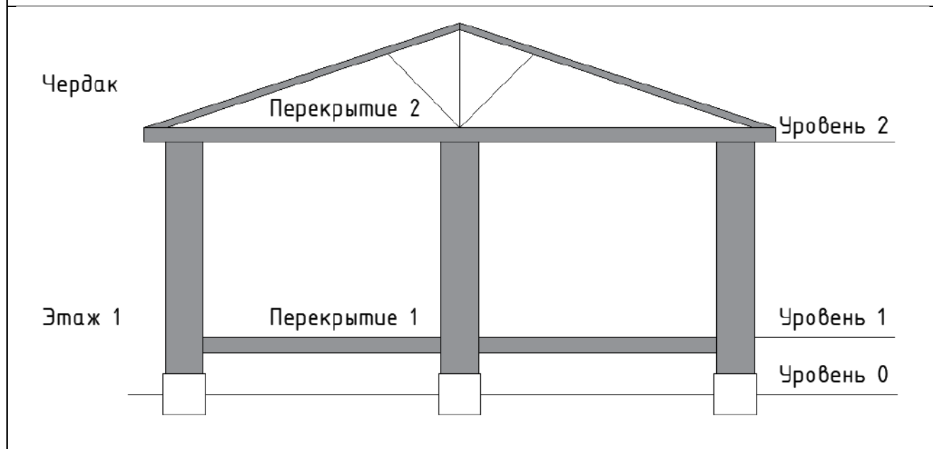
Схема разреза
