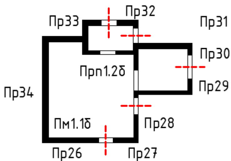
Б-Фасад 1 (фундамент 1, стена 1, покрытие 1)
