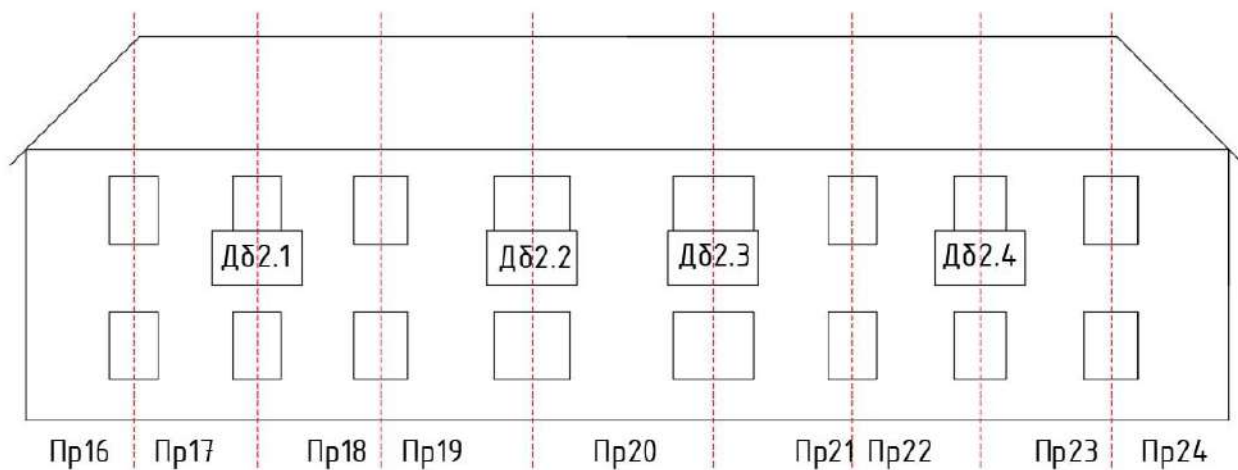
Фасад 3 (фундамент 3, стека 3, покрытие 3)
