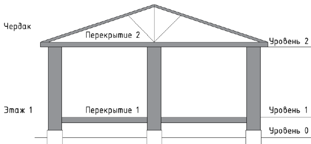
В-Схема разреза
