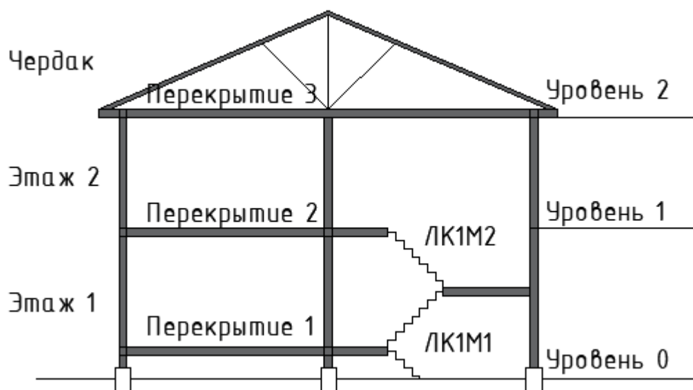
В-Схема разреза
