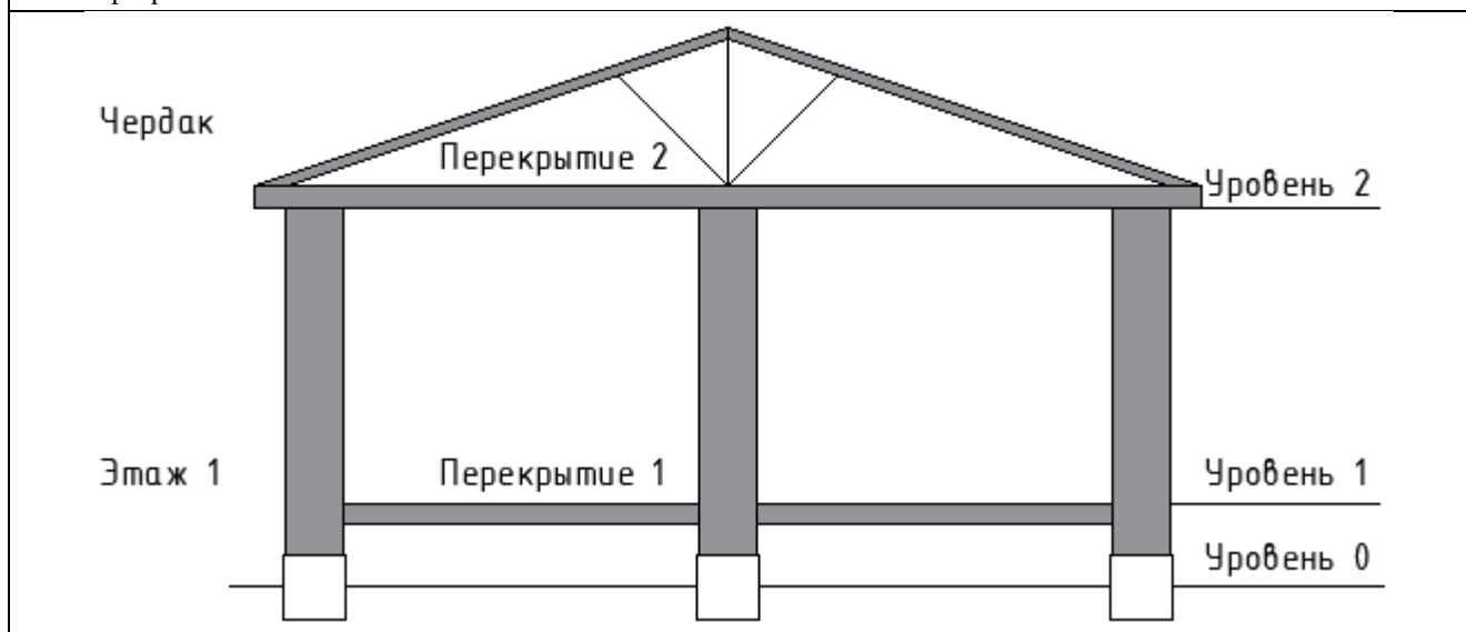
Схема разреза
