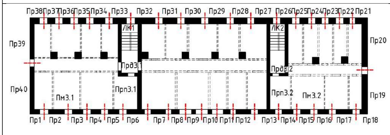
План 3-ого этажа
