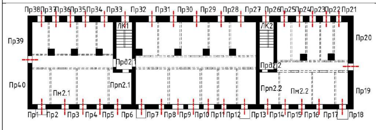
План 3-ого этажа
