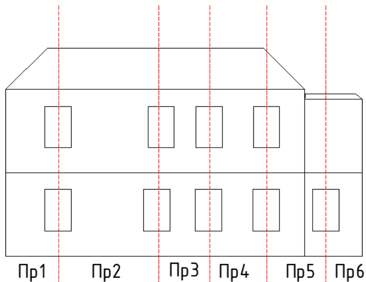
Фасад 2 (фундамент 2, стена 2, покрытие 2)
