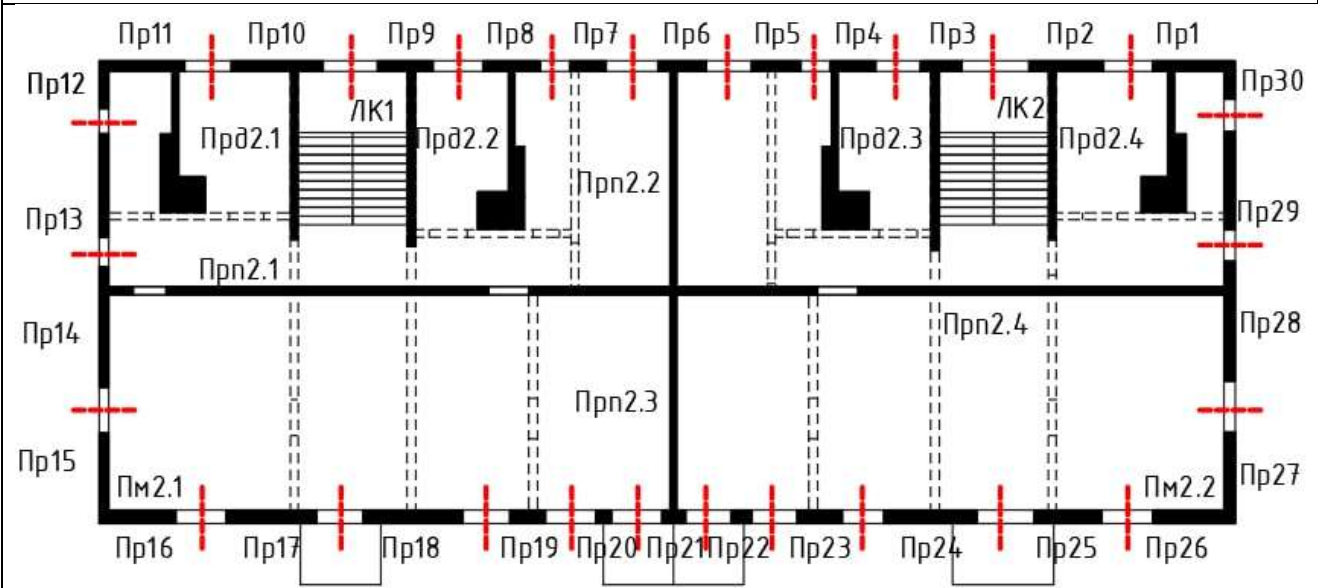
План 2-ого этажа
